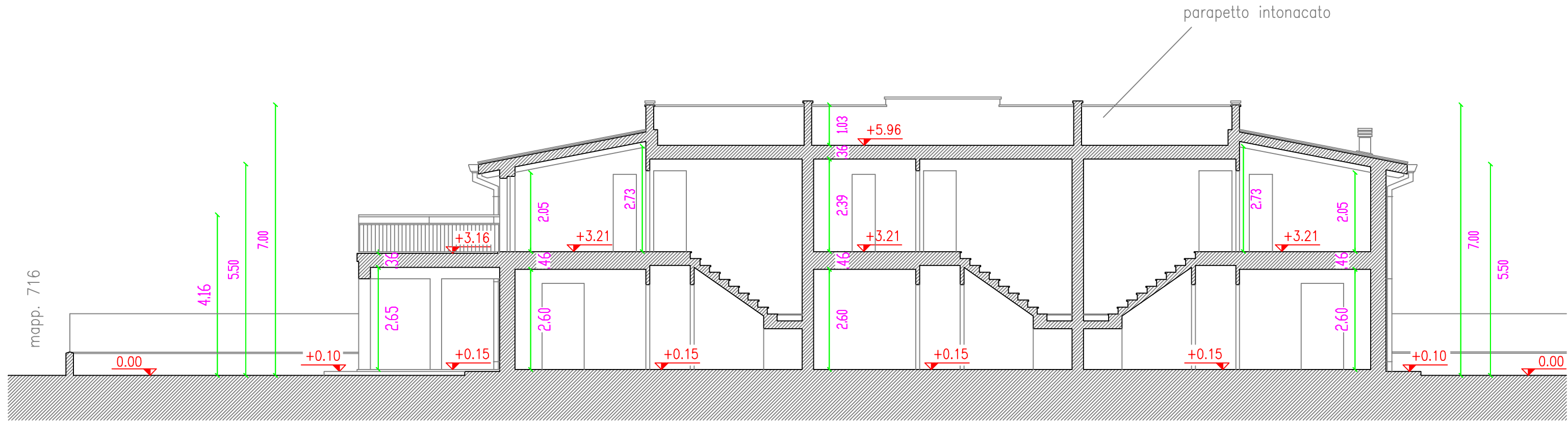
SEZIONE B
